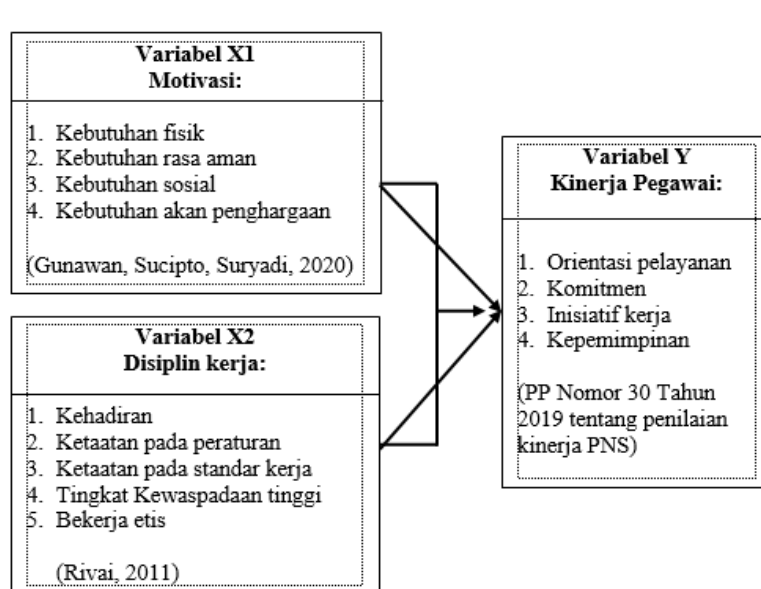
Gambar 1. Kerangka Pemikiran
