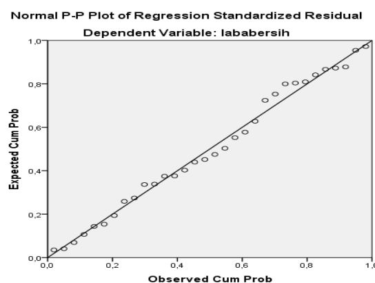
Gambar 1 Grafik normalitas
