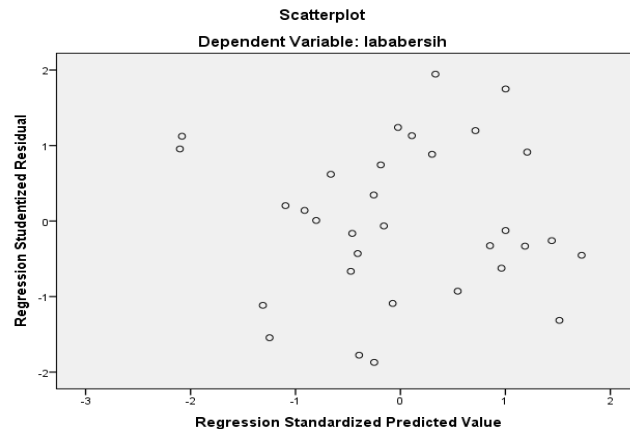
Gambar 2 Uji Heteroskedastisitas
