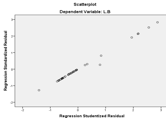
Gambar 2 Grafik Heteroskedastisitas
